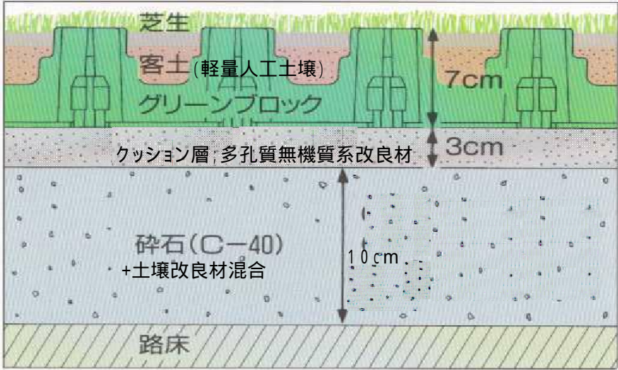
断面図
